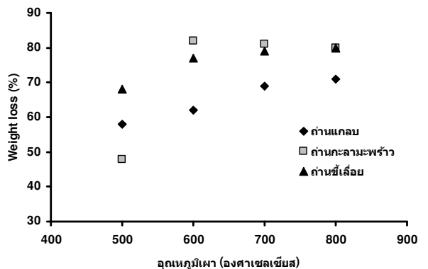
รูปที่ 1 Weight loss, ปริมาณที่หายไปของถ่านชนิดต่างๆ ต่ออุณหภูมิที่ใช้เป็นเวลา 3 ชั่วโมง
