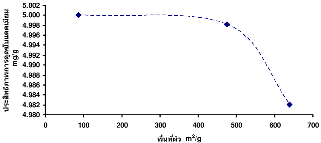
รูปที่ 5 ความสัมพันธ์ระหว่างประสิทธิภาพการดูดซับแคดเมียมต่อพื้นที่ผิวของถ่าน
