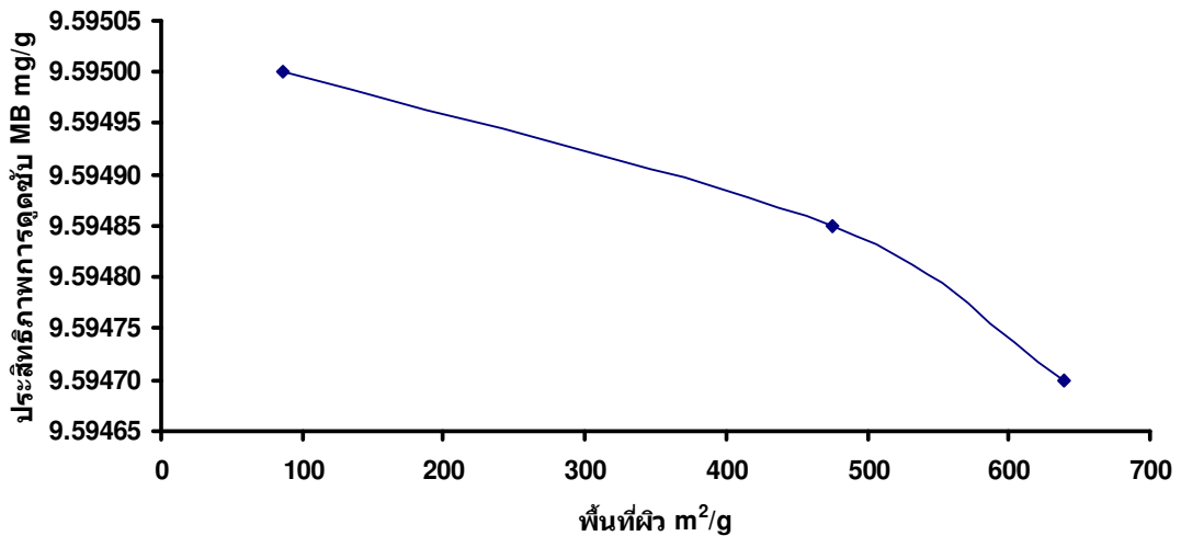
รูปที่ 4 แสดงประสิทธิภาพการดูดซับสีของ Methylene blue ต่อพื้นที่ผิวของถ่าน
