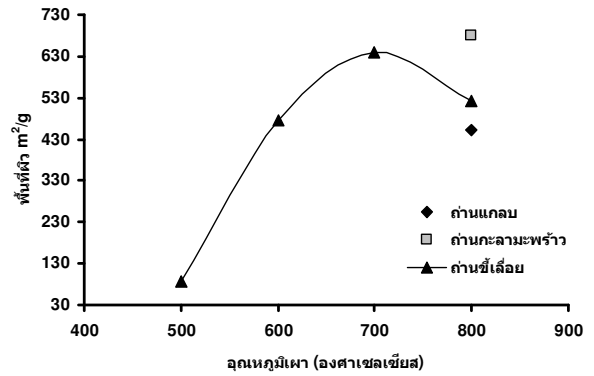
รูปที่ 2 พื้นที่ผิวของถ่านจี้เลื่อย แกลบ และกะลามะพร้าว ต่ออุณหภูมิที่ใช้เผา
